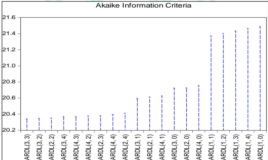
الشكل (٣) فترات الابطاء المثلى
